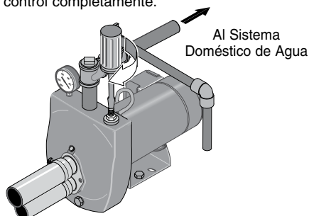
Figura 13: Cebado de la Bomba
