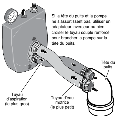
Figure 2 : Branchement inversé dans le puits
