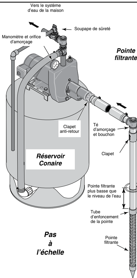
Figure 5 : Installations typiques dans un puits peu profond
