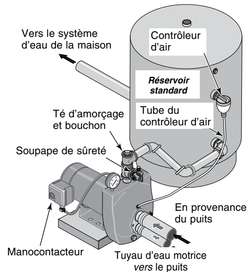
Figure 7 : Branchements sur un réservoir standard
