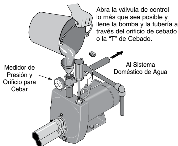
Figura 12: Llenado de la Bomba
