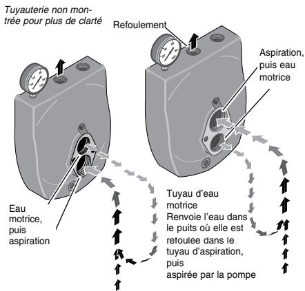
Figure 1 : Fonctions eau motrice et aspiration
