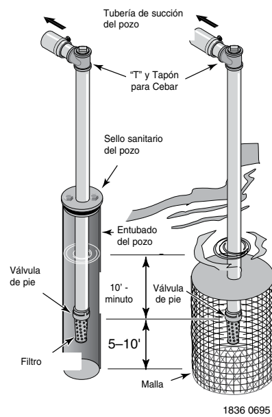
Figura 5: Instalación típica para pozo poco profundo
