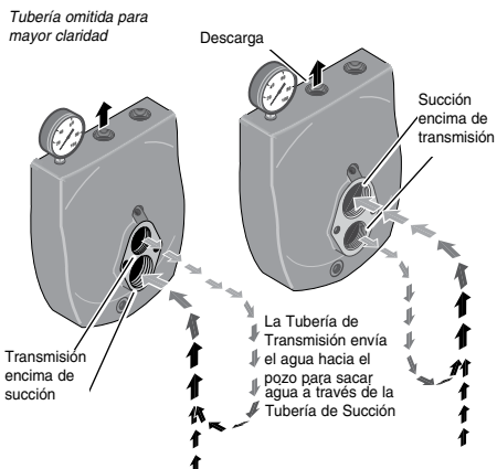
Figura 1: Funciones de Succión y Transmisión
