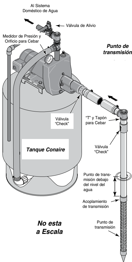
Figura 5: Instalación típica para pozo poco profundo
