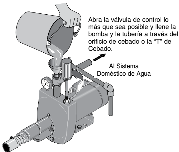
Figura 15: Abrir la Válvula de Control
