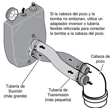
Figura 2: Conexiones Invertidas hacia el Pozo
