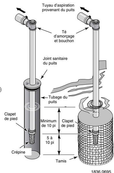
Figure 5 : Installations typiques dans un puits peu profond
